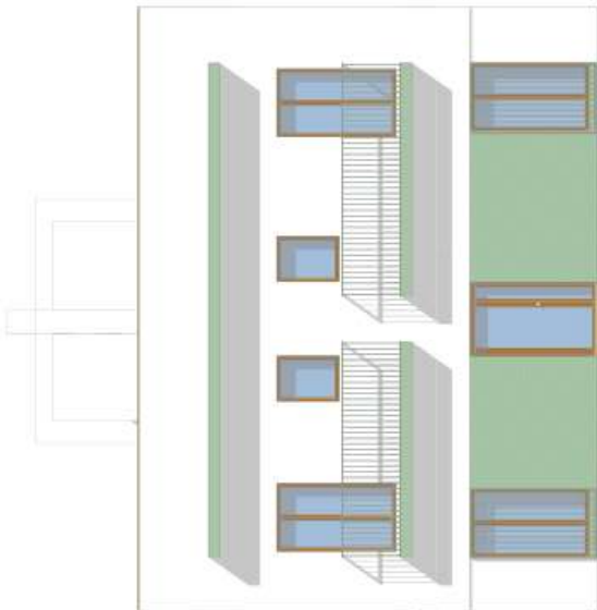
ALZADO EXTERIOR
