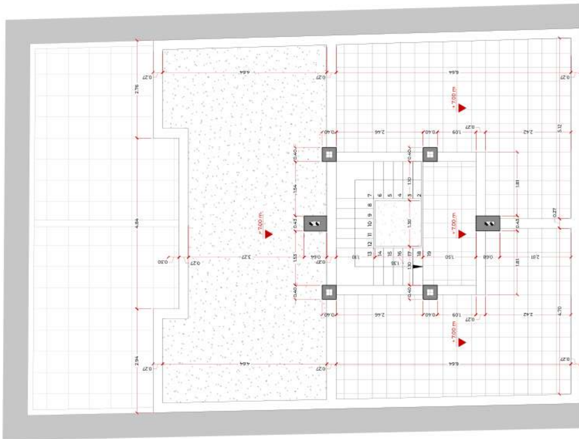
PLANTA CUBIERTA
