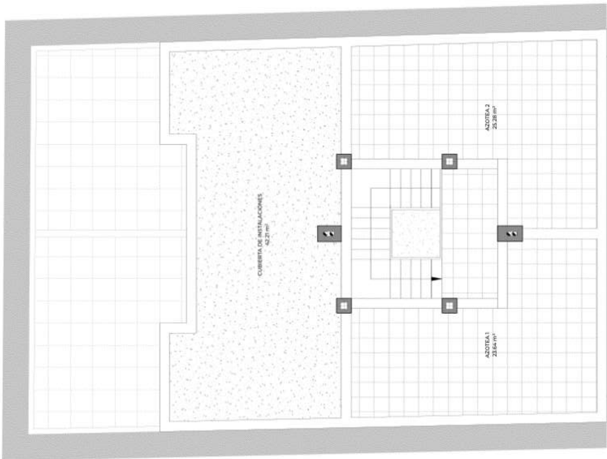
PLANTA CUBIERTA
