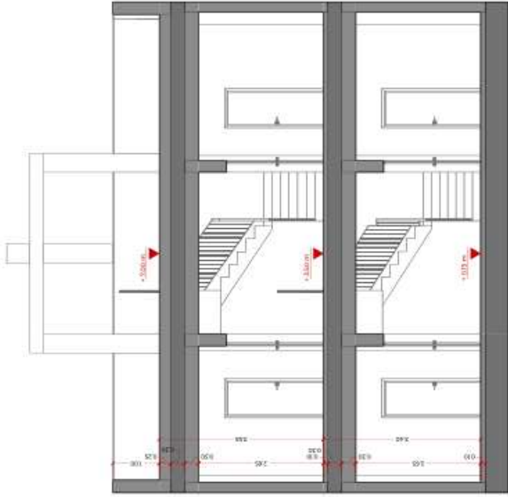
SECCIÓN I
